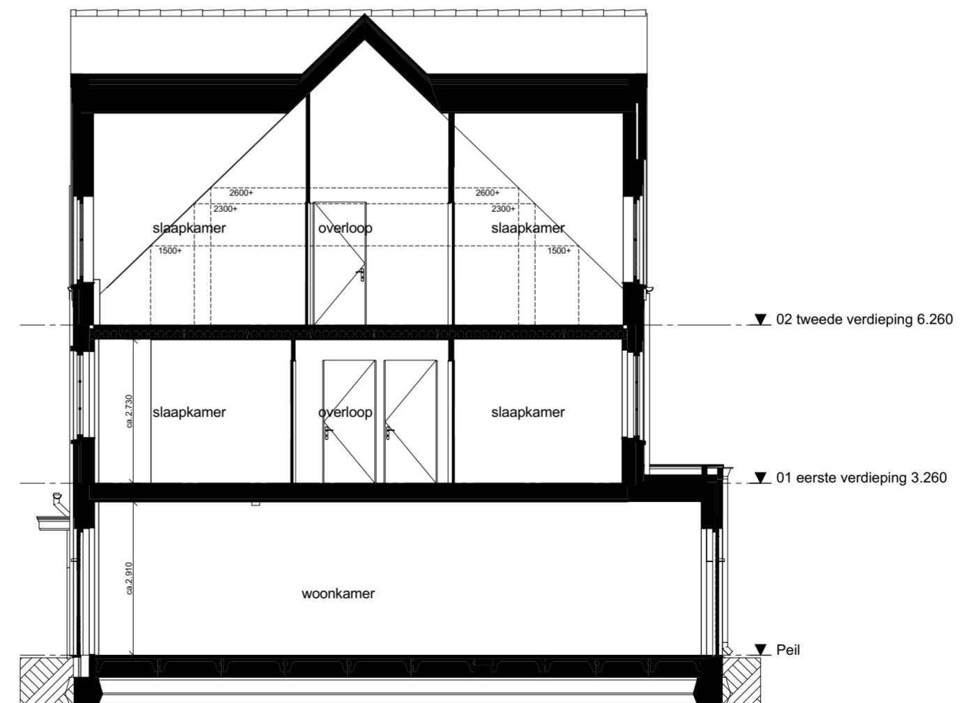
Doorsnede A-A L2b 1:100
