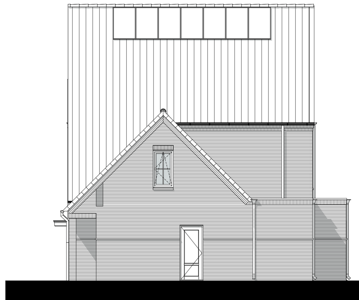
Rechtergevel 1:100
