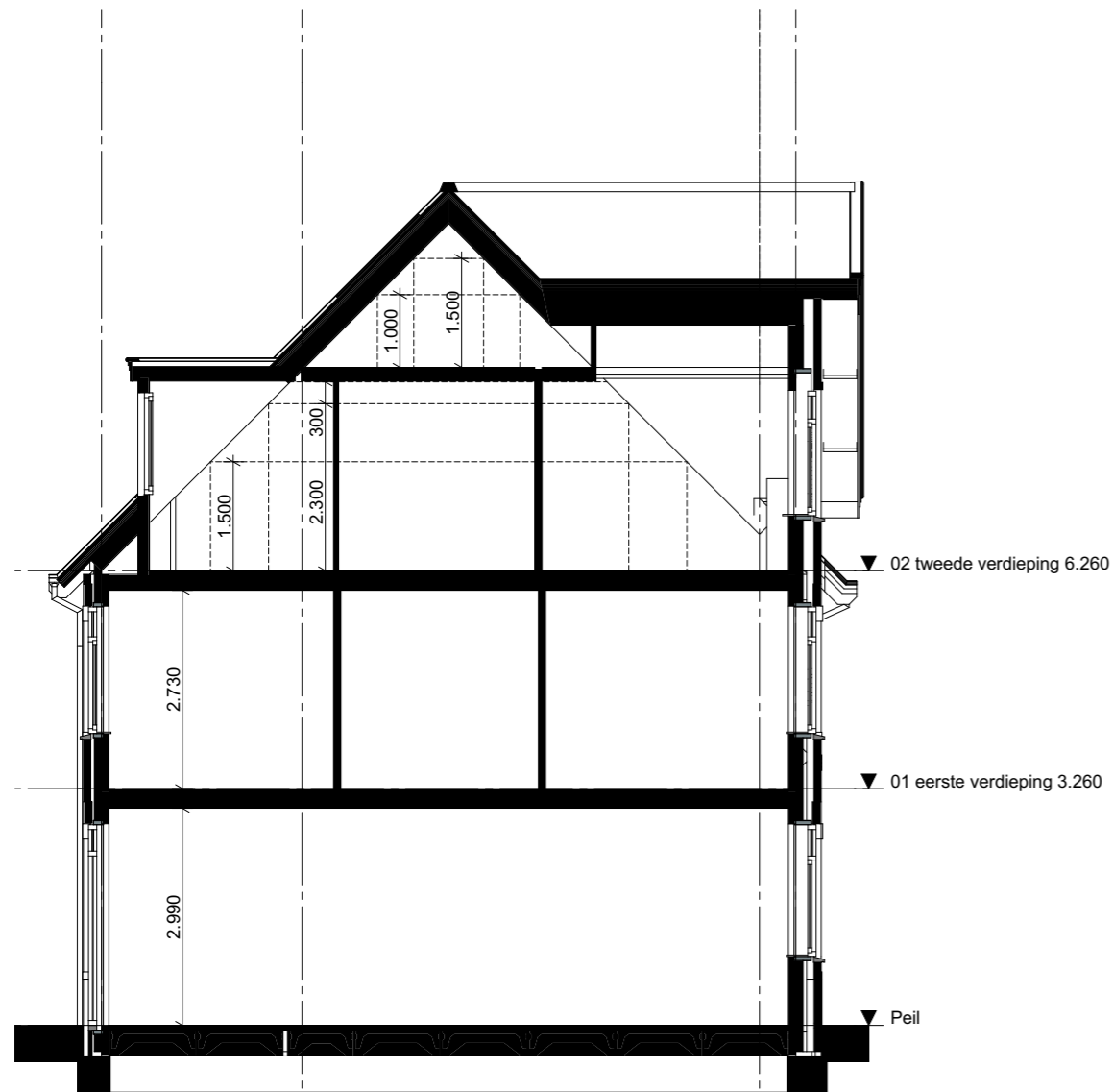
Doorsnede B1-B1
