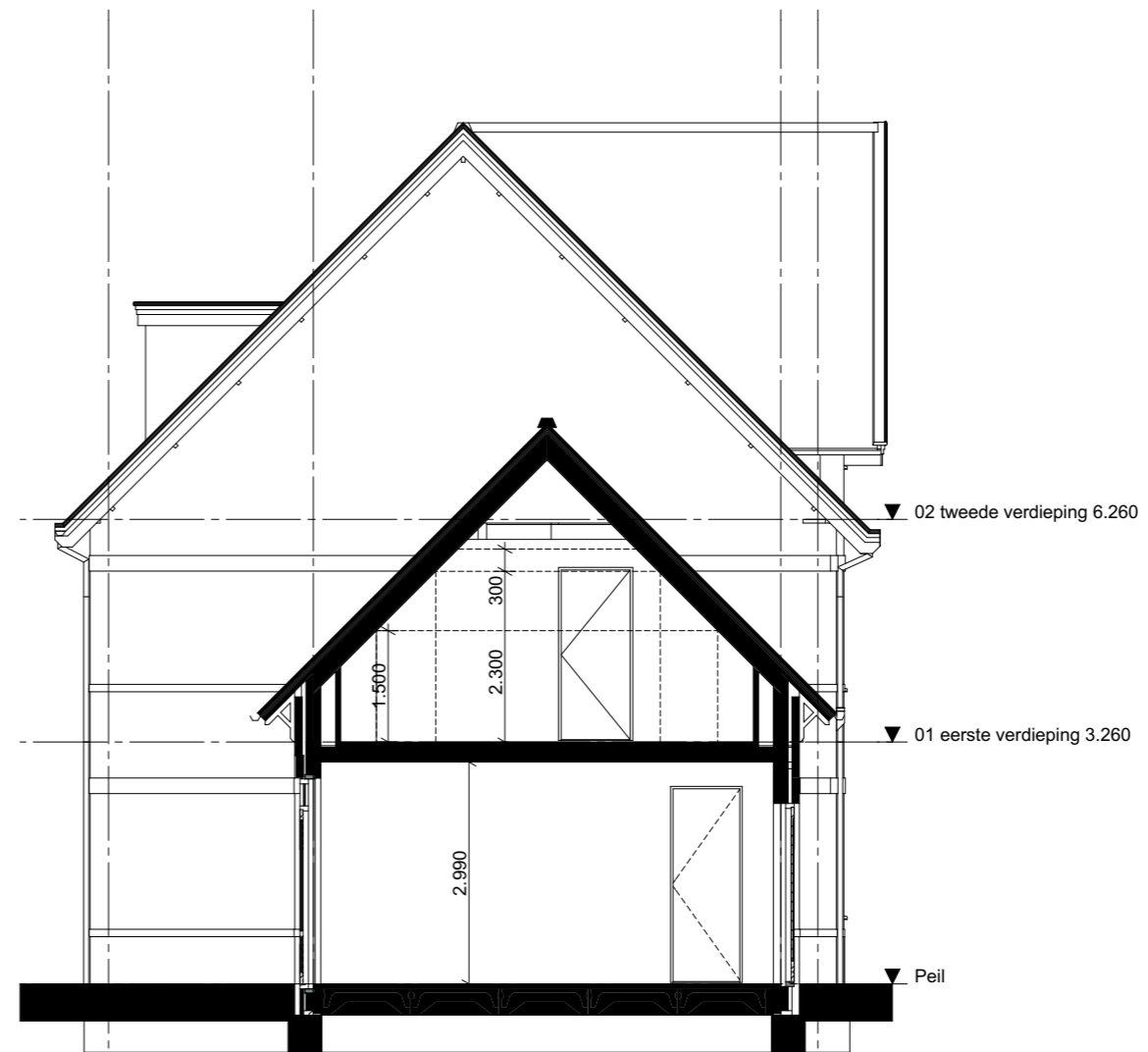
Doorsnede C1-C1
