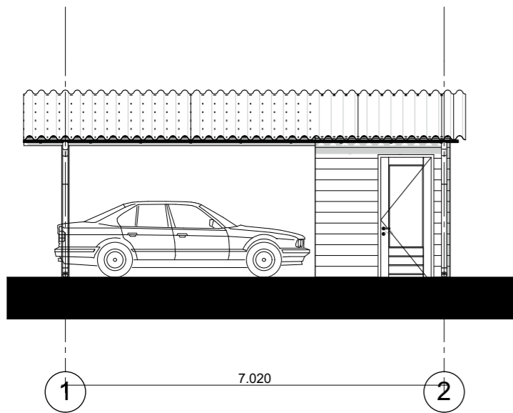
Voorgevel 1:100
