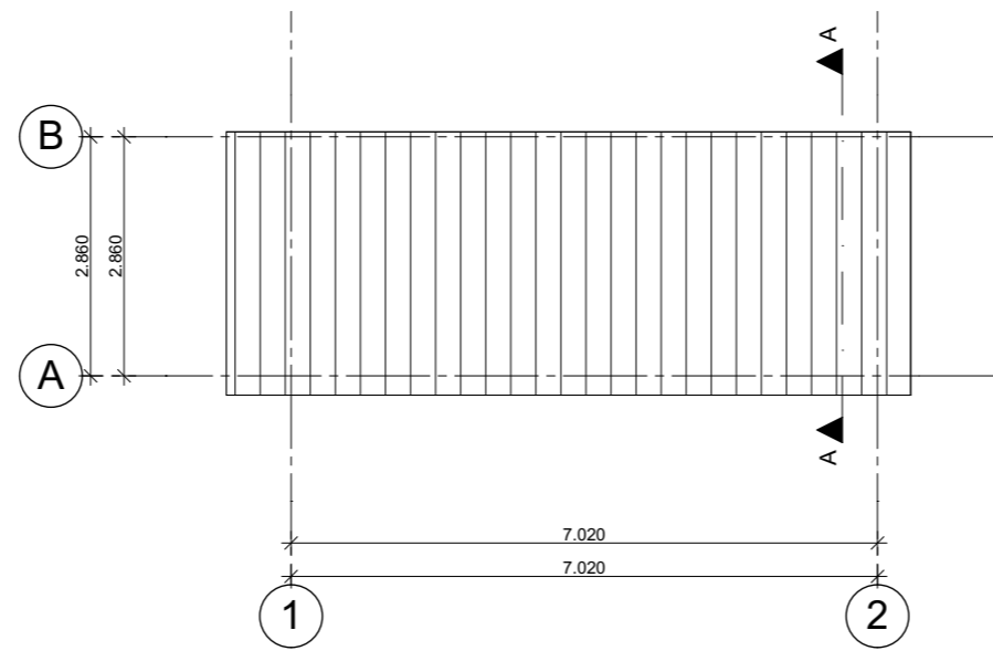
dak 1:100
