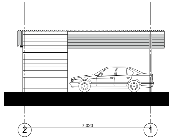
Achtergevel 1:100
