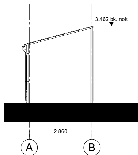
Doorsnede A-A 1:100
