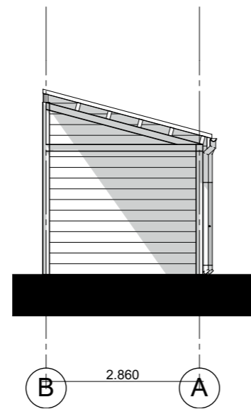
Linkergevel 1:100
