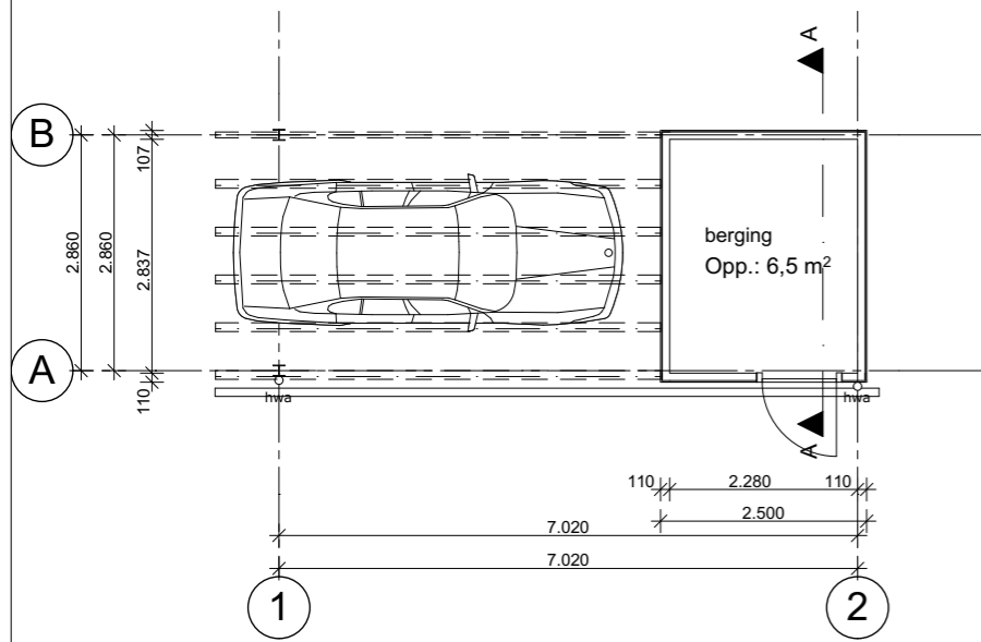
Begane grond 1:100
