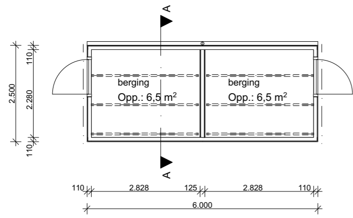
Begane grond 1:100
