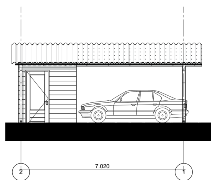
Linkergevel 1:100
