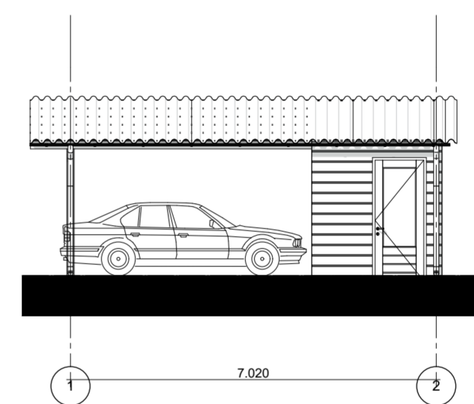
Rechtergevel 1:100
