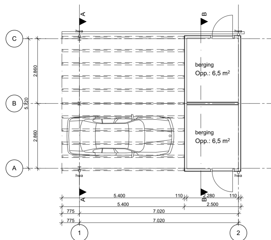
Begane grond 1:100
