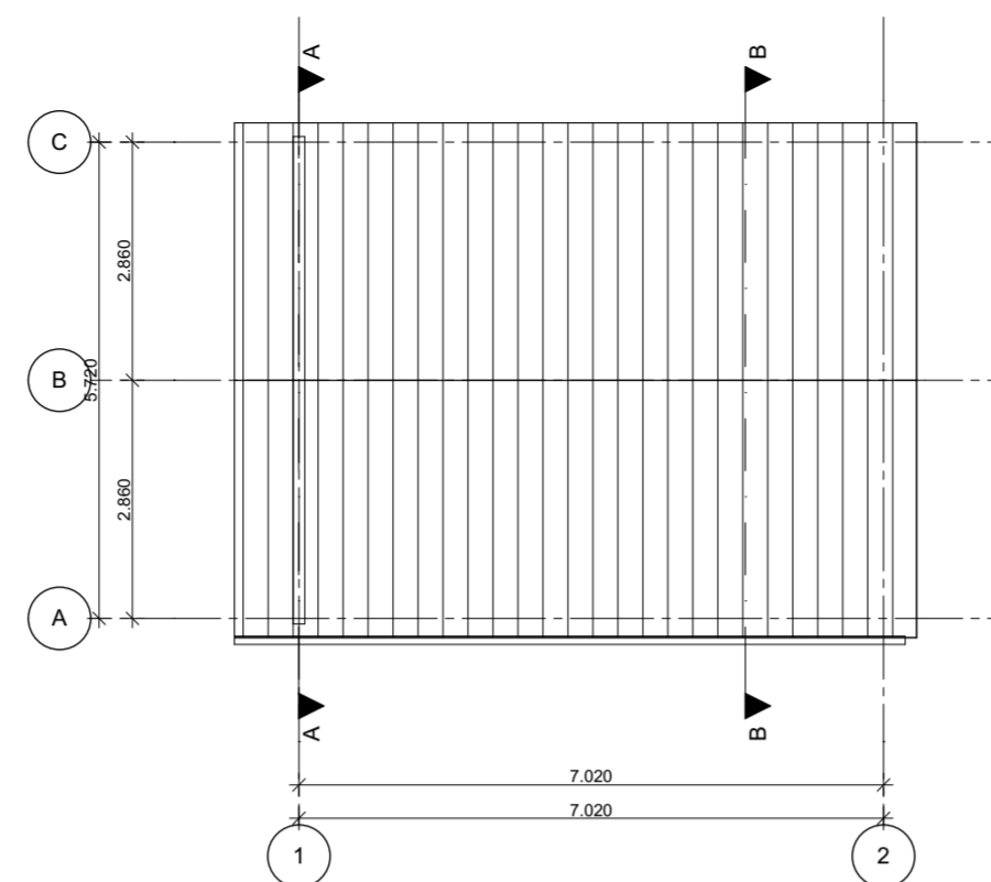
dak 1:100
