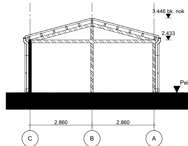
Doorsnede A-A 1:100
