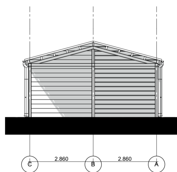
Voorgevel 1:100
