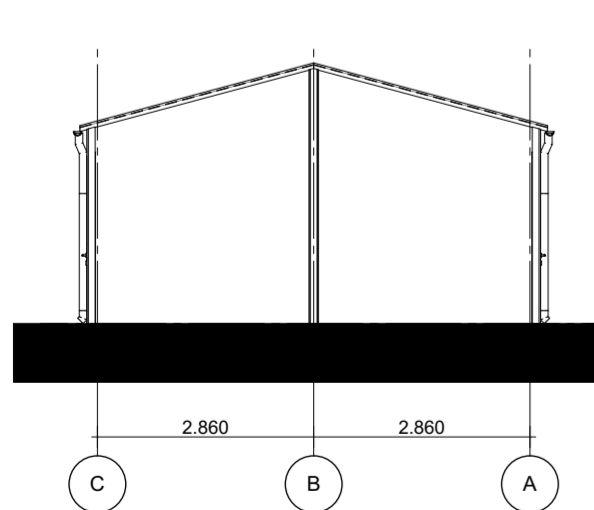
Doorsnede B-B 1:100
