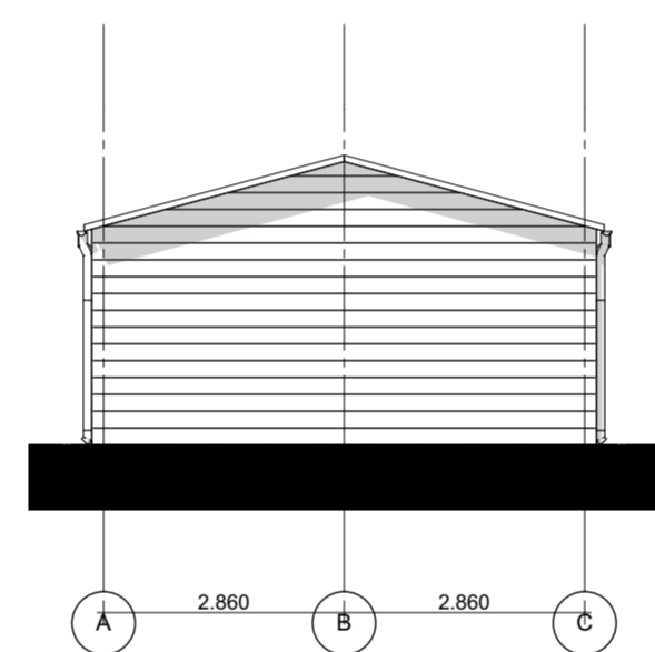
Achtergevel 1:100
