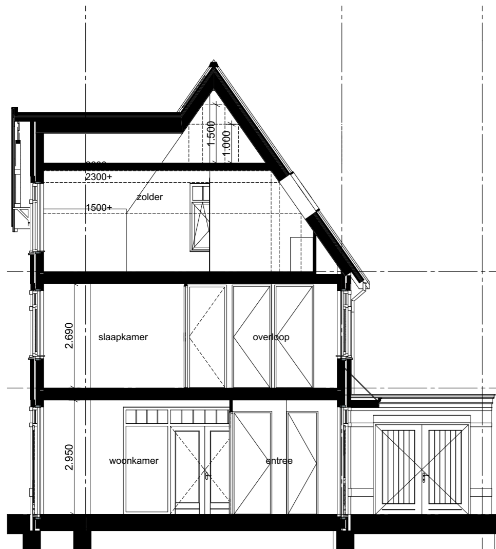
Doorsnede A-A
