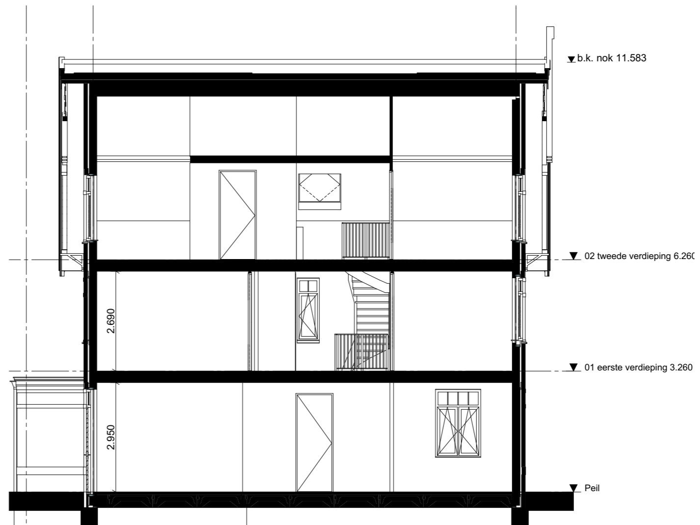
Doorsnede B-B
