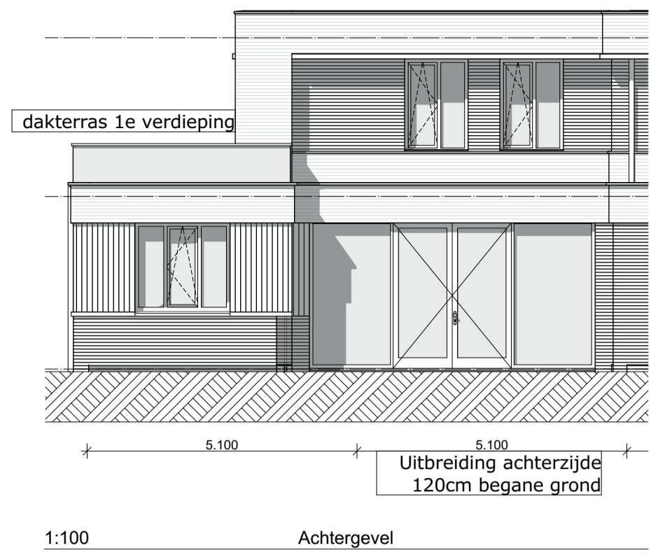
1:100 Achtergevel
