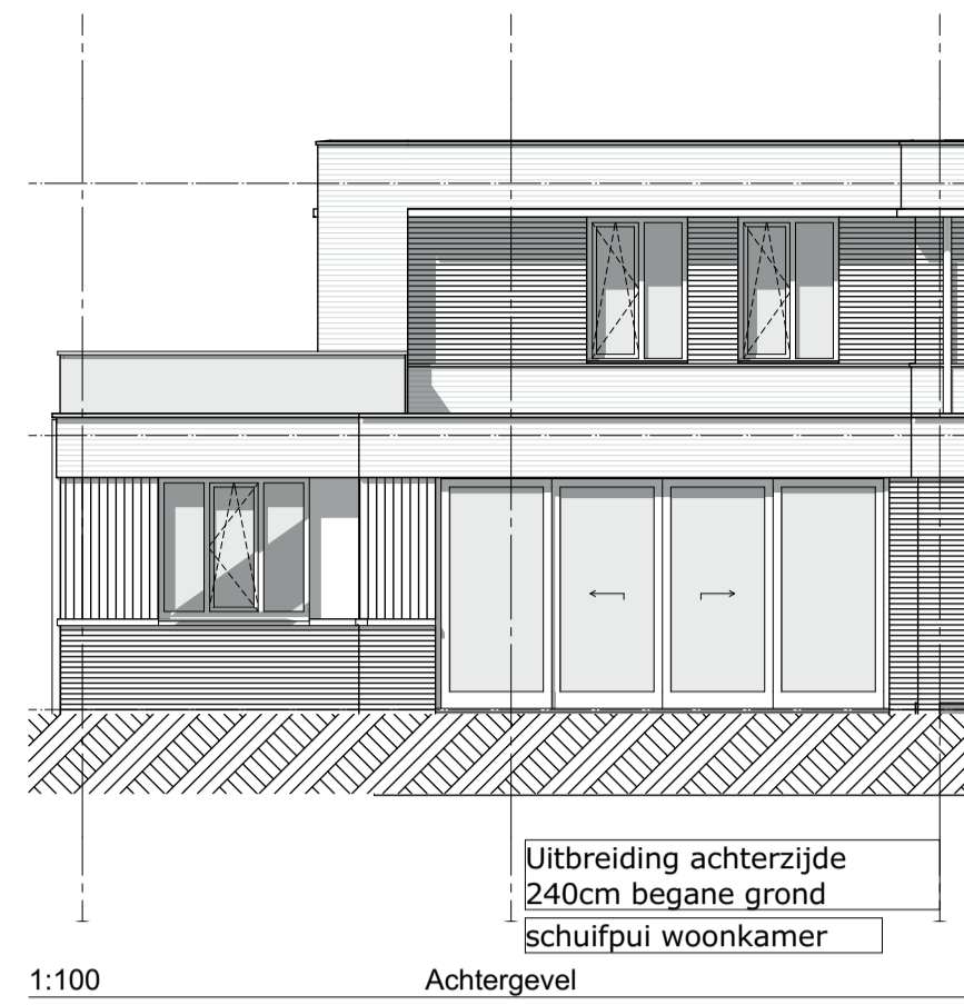
1:100 Achtergevel
