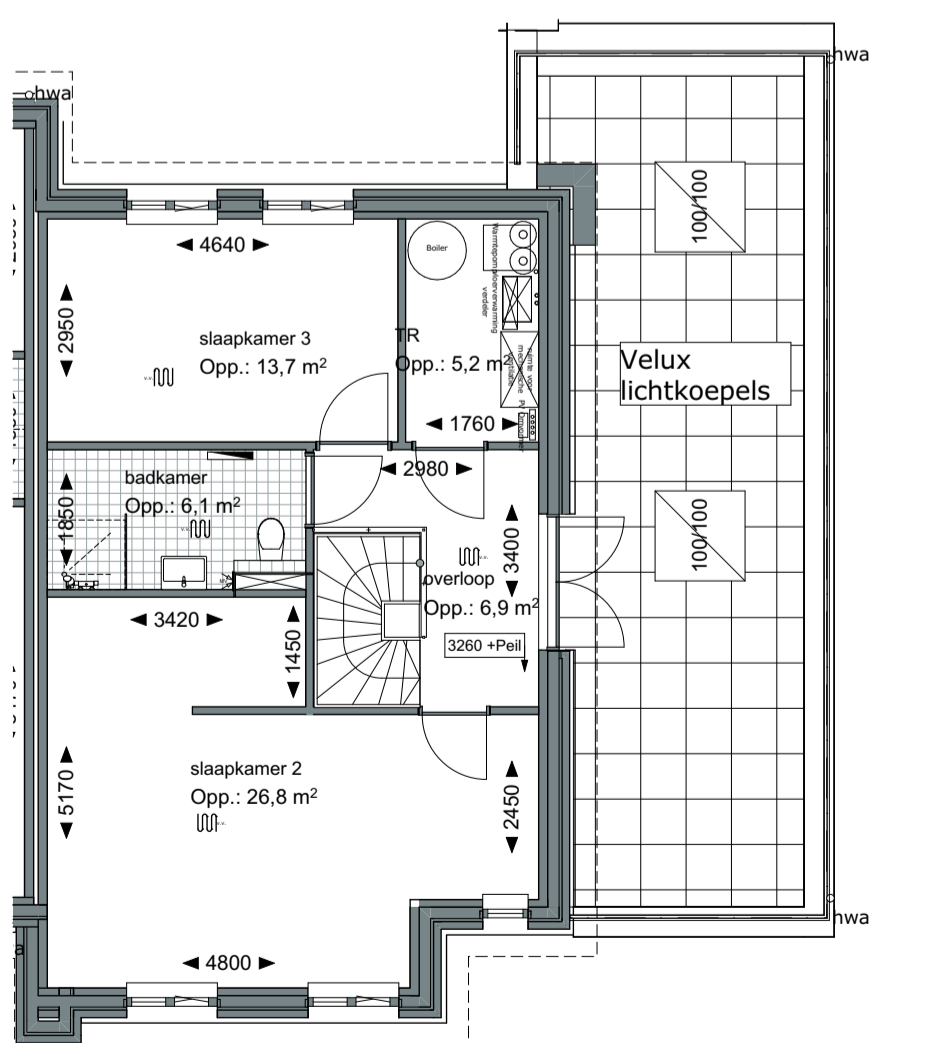
1:100 01 eerste verdieping
