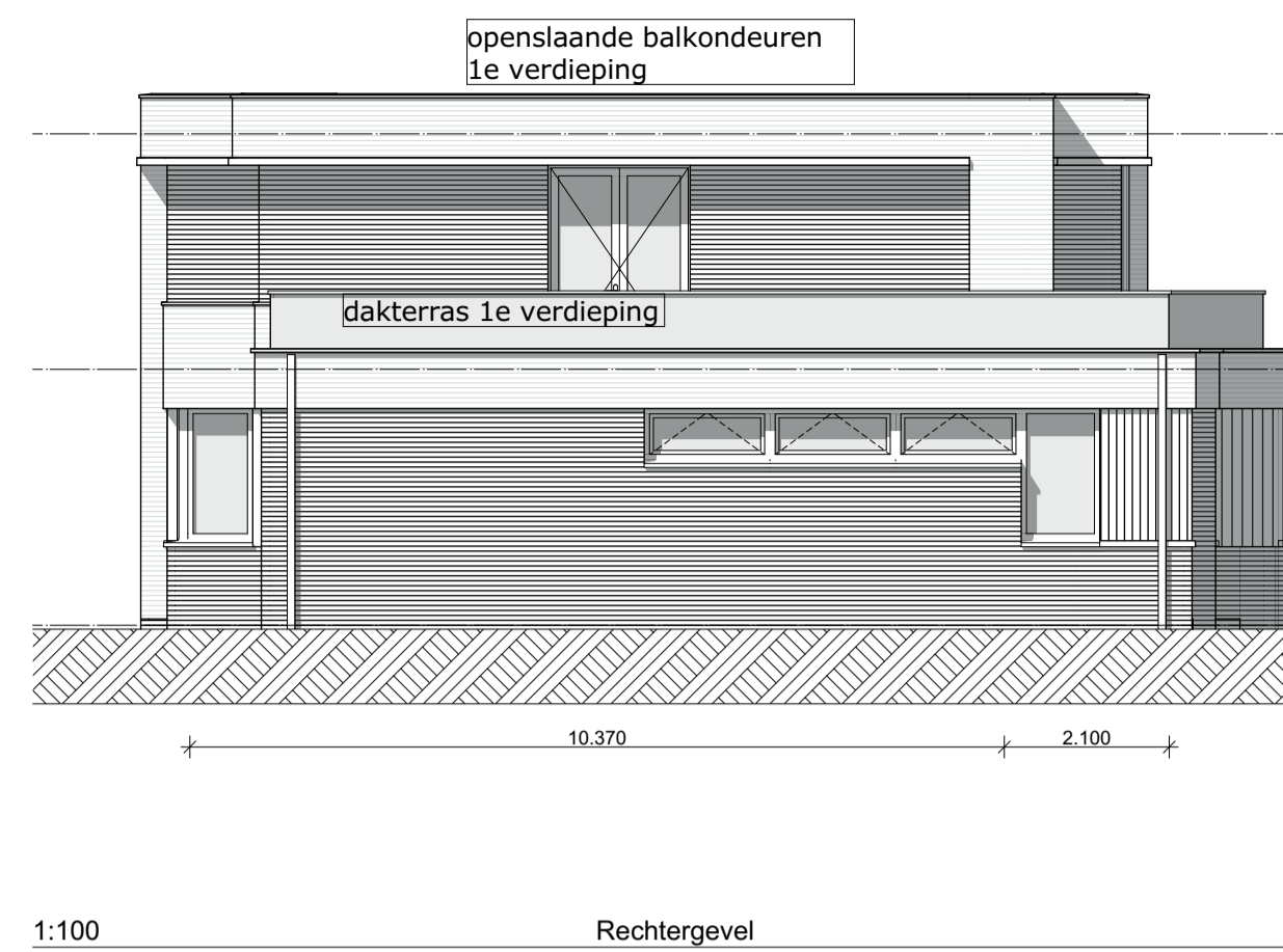
1:100 Rechtergevel
