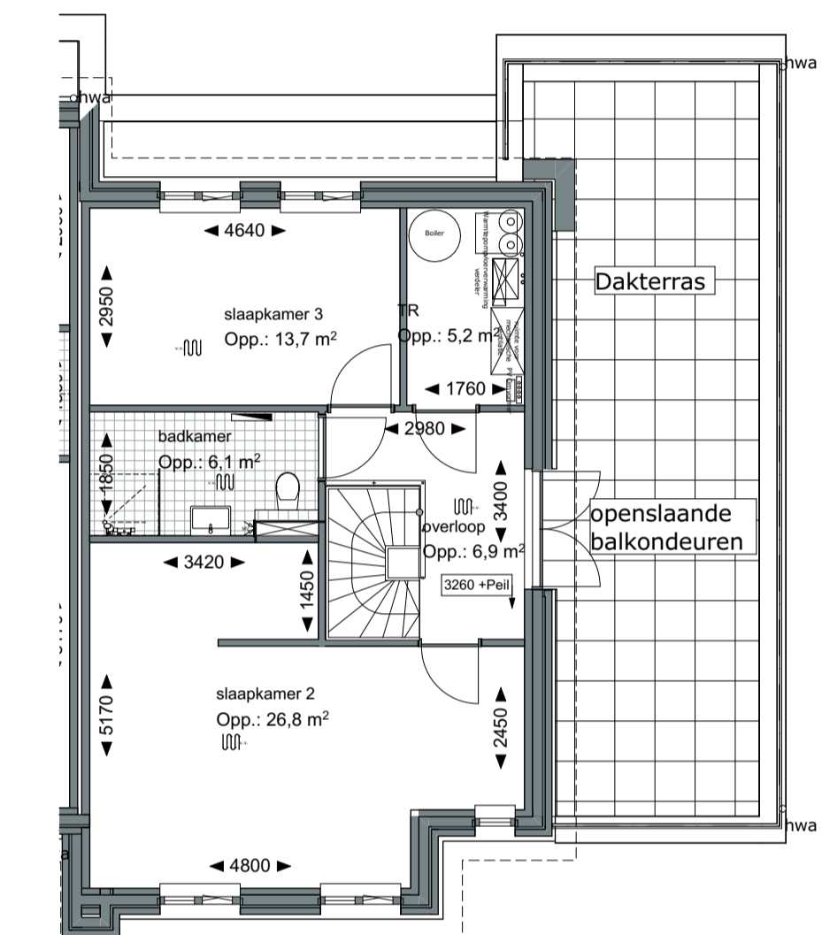
1:100 01 eerste verdieping
