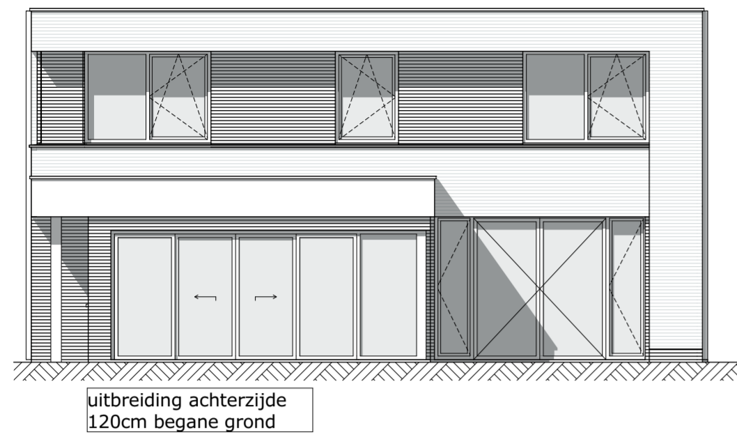
1:100 Achtergevel
