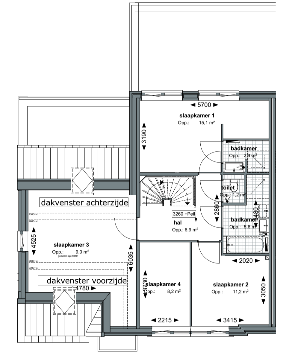
1:100 01 eerste verdieping
