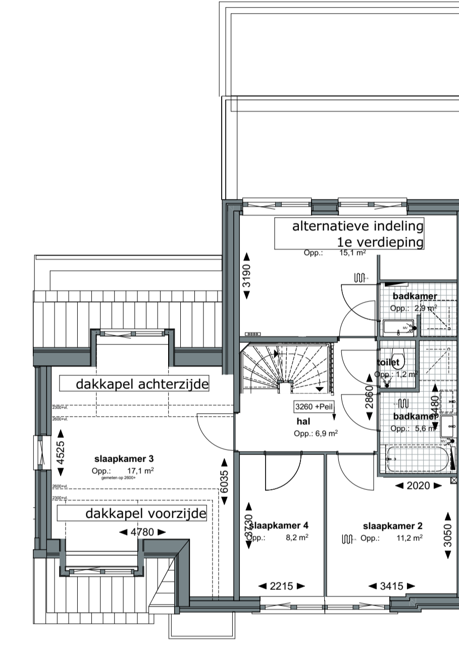
1:100 01 eerste verdieping
