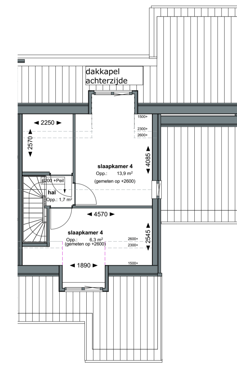
1:100 02 2e verdieping
