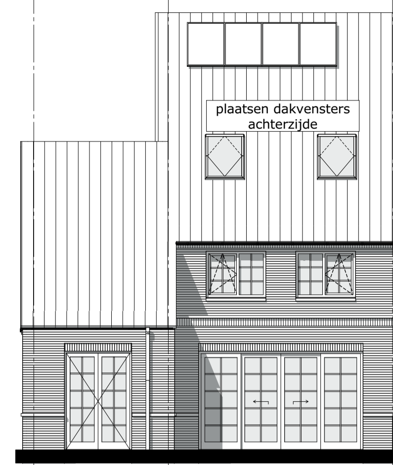
1:100 Achtergevel
