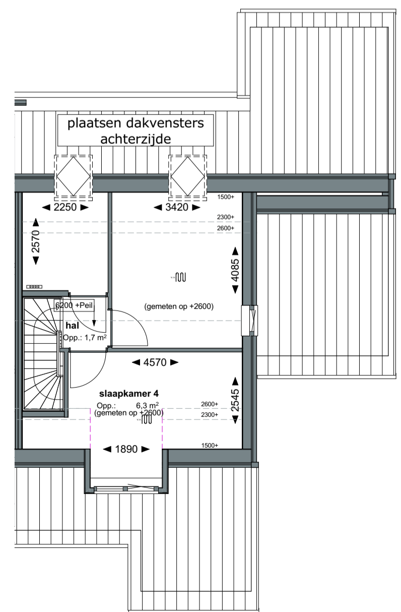
1:100 02 2e verdieping
